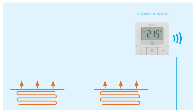
Riadiaca stanica podlahového vykurovania - max. 6 zón
