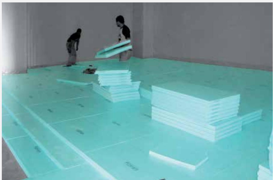
Tepelnoizolačné dosky FIBRANxps 300-L s rovnou hranou sú určené na použitie vo viacerých vrstvách.
